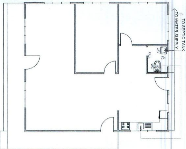
PLUMBING LAYOUT SCALE: 1:100
